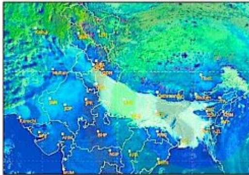
उपग्रह से प्राप्त चित्र में उत्तर भारत के राज्यों पर कोहरे की मोटी चादर दिख रही है।
